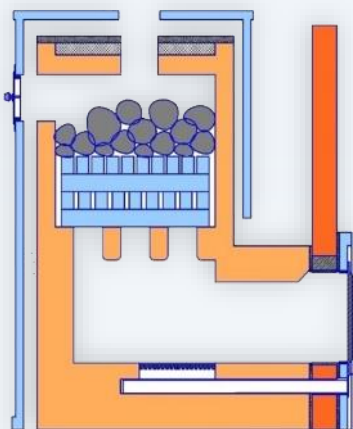
Печь для Бани По-Серому
