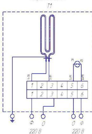
Электрическая схема электрокаменки ANNIKKI Навесная Н1 с одним ТЭНом мощность 12 кВт, напряжение 220 В
