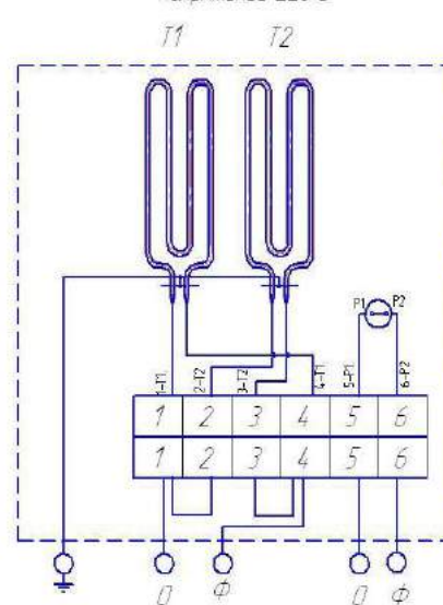
Электрическая схема электрокаменки ANNICKI Навесная Н2 с двумя ТЭНами общей мощностью 24 кВт, напряжение 220 В
