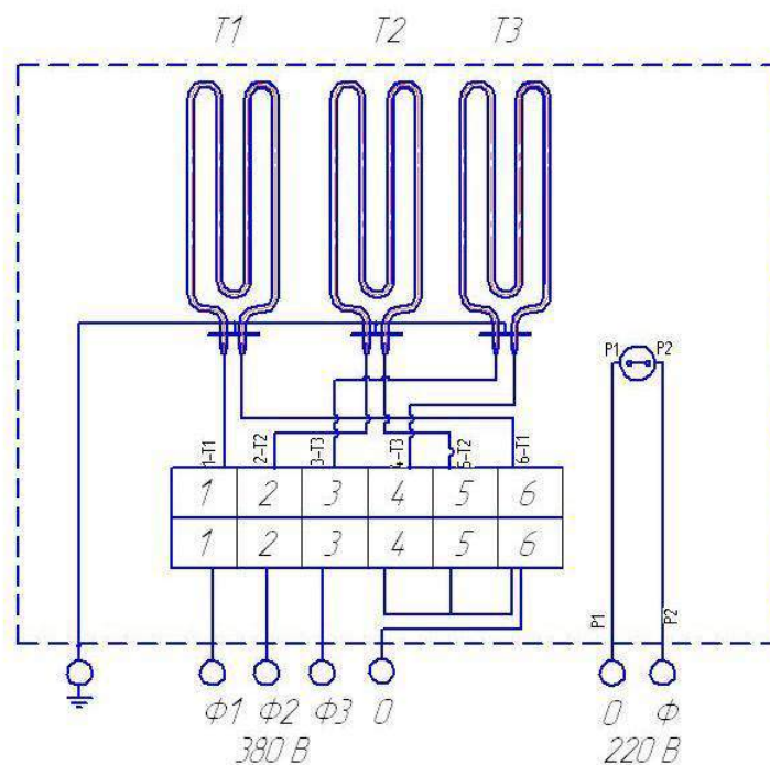
Электрическая схема электрокаменки ANNICKI Навесная Н3 с тремя ТЭНами общей мощностью 3,6 кВт, напряжение 380 В
