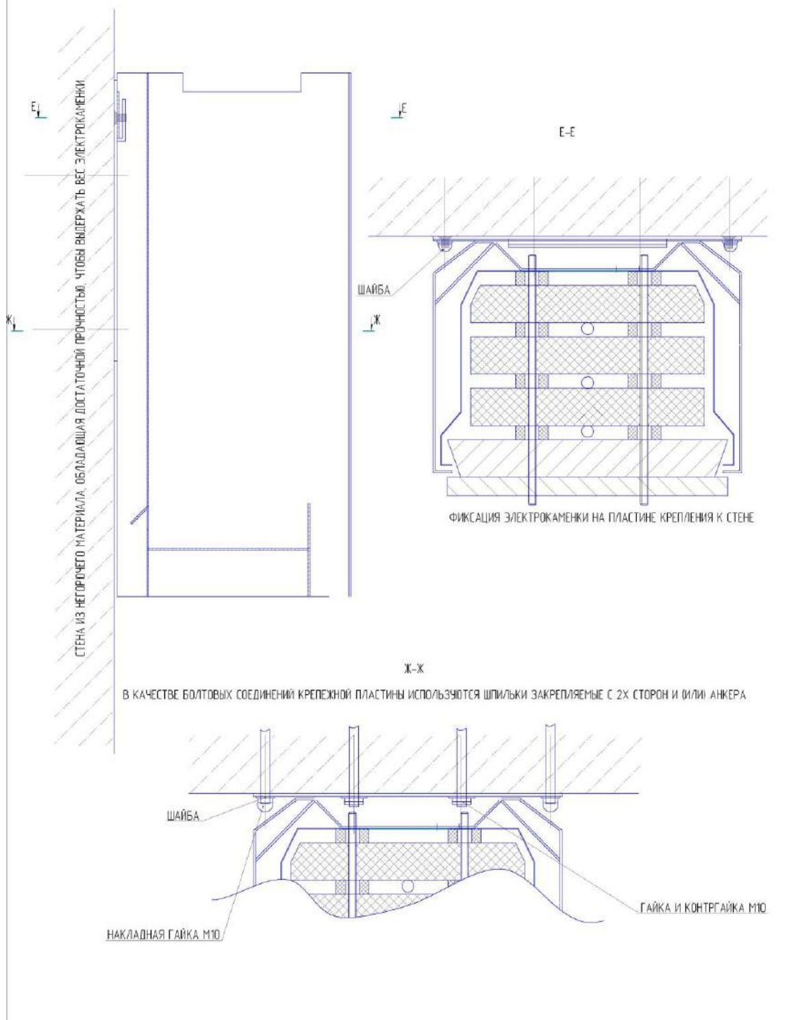
Схема установки на пластину крепления электрокаменки ANNIKKI Навесная
